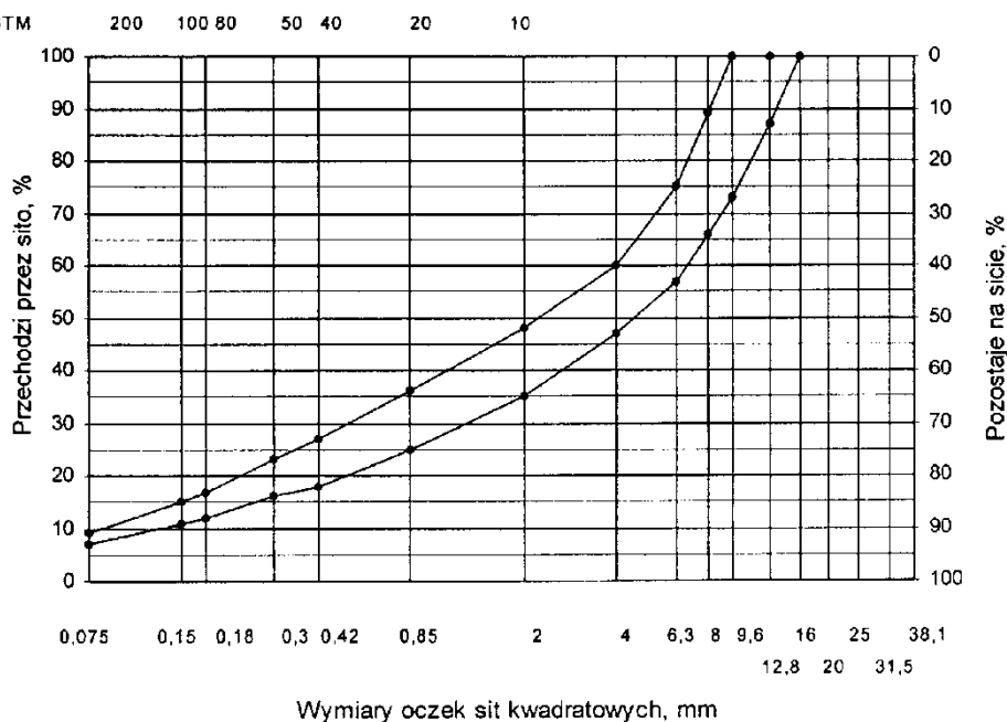
Rys. 7. Krzywe graniczne uziarnienia mieszanki mineralnej BA od 0 do 12,8 mm do warstwy ściernawej nawierzchni drogi o obciążeniu ruchem od KR3 do KR6
