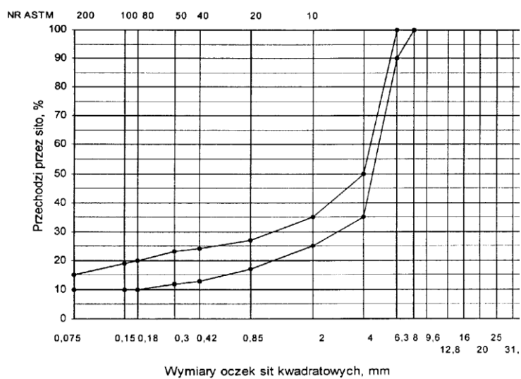
Rys. 3. Krzywe graniczne uziarnienia mieszanki mineralnej SMA od 0 do 6,3 mm do warstwy ścieralnej nawierzchni drogi o obciążeniu ruchem KR1 lub KR2
