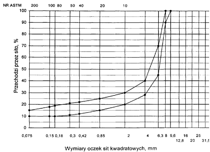
Rys. 2. Krzywe graniczne uziarnienia mieszanki mineralnej SMA od 0 do 8 mm do warstwy ścieralnej nawierzchni drogi o obciążeniu ruchem KR1 lub KR2
